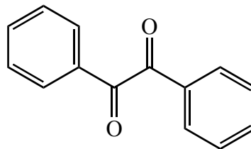
benzil (mp 96°)
