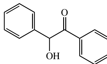
benzoin (mp 133°)
