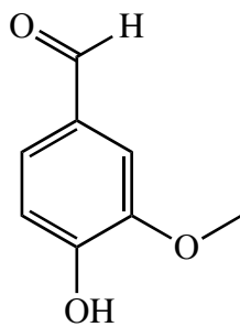
vanillin (mp 81°)
